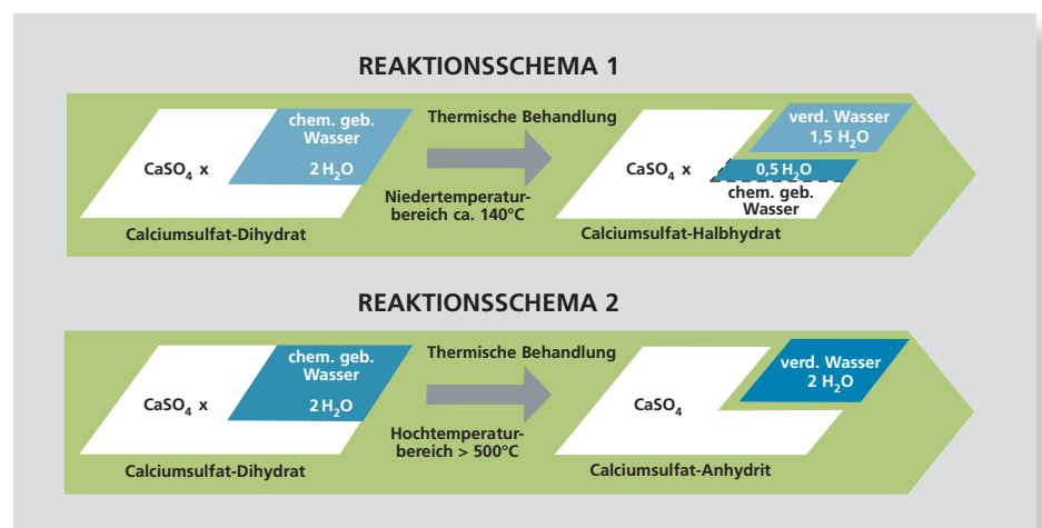
Abb. 1: Die Bildung von Calciumsulfat-Halbihydrat (1) und von Calciumsulfat-Anhydrit (2) aus Calciumsulfat-Dihydrat
