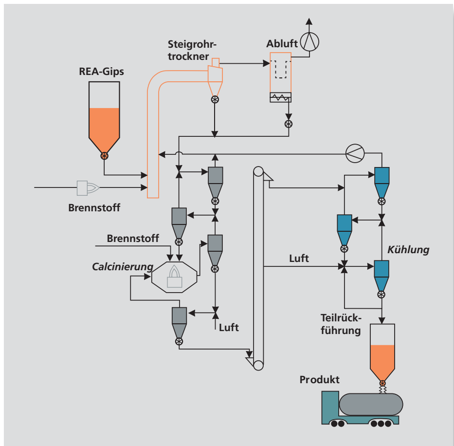
Abb. 12: Die Bildung von Thermischem Anhydrit aus REA-Gips
