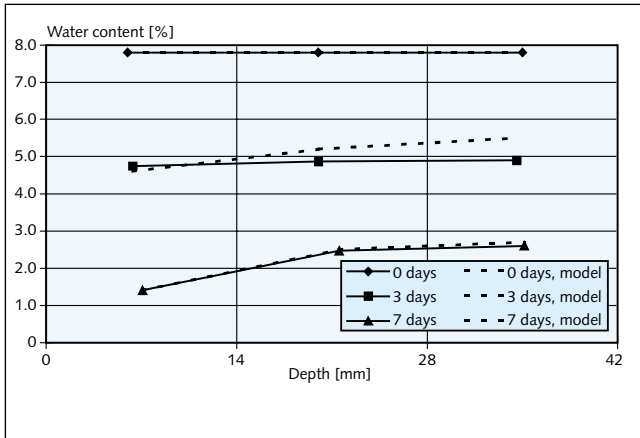
4 Gravimetrisch bestimmte sowie berechnete Feuchtegradienten für 42 mm dicke Probekörper 4 Gravimetrically determined and calculated moisture gradients for the 42 mm thick test piece
